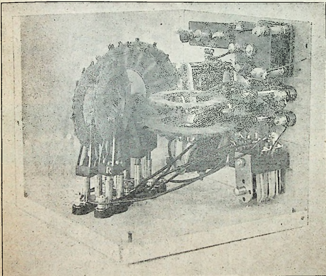
Spoelstel I inwendig (2 wanden zijn weggenomen). Foto G. J. Eschauzier.
